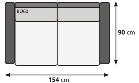
2 zit (ARM1L + BO60 + ARM1R)
